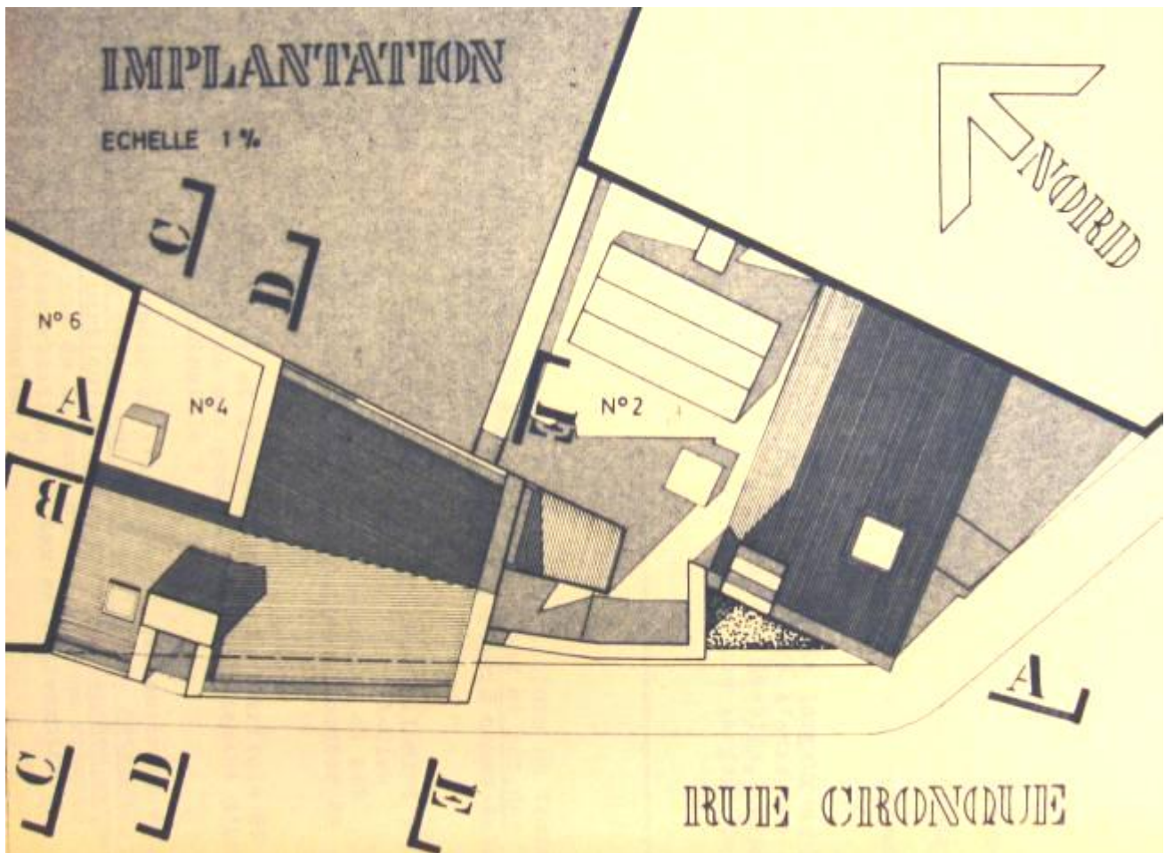
Figure 01 : maison de l'architecte André Godart., rue Cronque 2-4, 7000 Mons, 1974-1975. Implantation (Archives de l'auteur)
